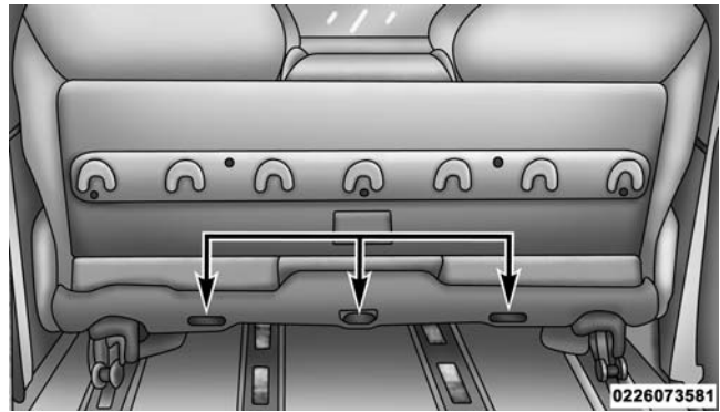
Ancrages de courroie d'attache de la banquette de troisième rangée
