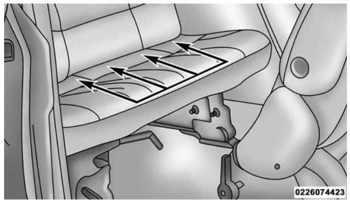
Ancrages inférieurs du système LATCH de banquette de 3 e rangée
