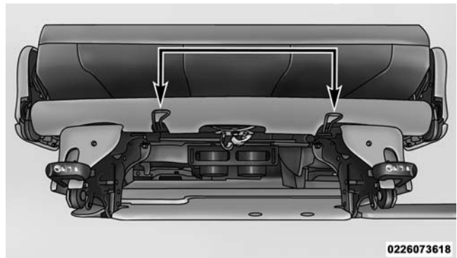
Ancrages de courroie d'attache de la banquette de deuxième rangée
