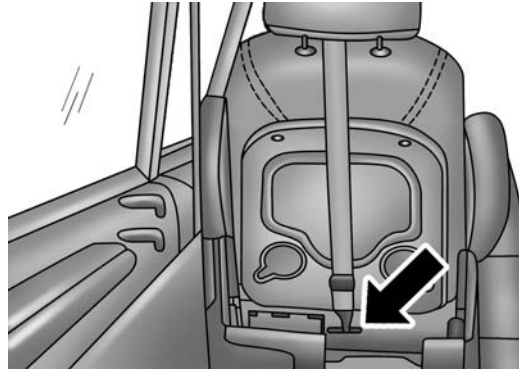
Ancrage de courroie d'attache du siège baquet de deuxième rangée
